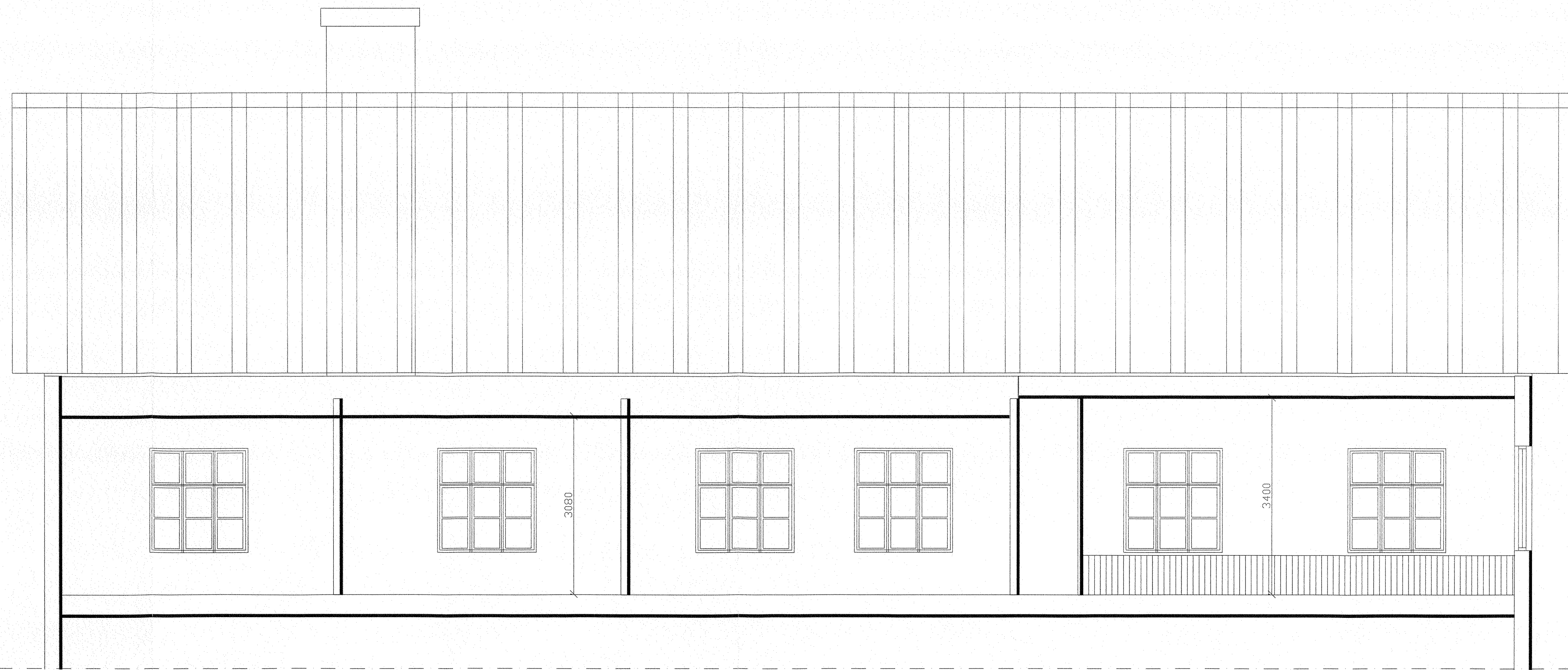
LEIKKAUS B-B
